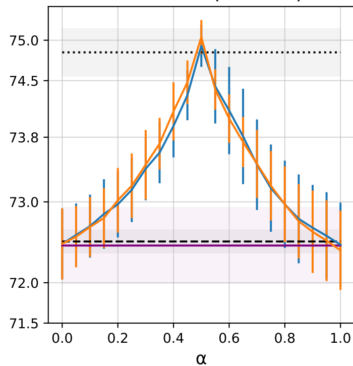
CIFAR100 (VGG16)
